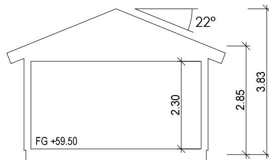
Sektion A-A
