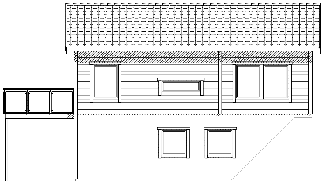
Fasad 3
