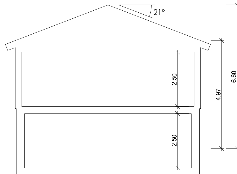
Sektion A-A
