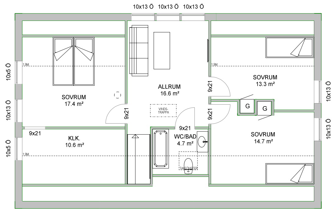
Överplan BOA 69.3 m²
