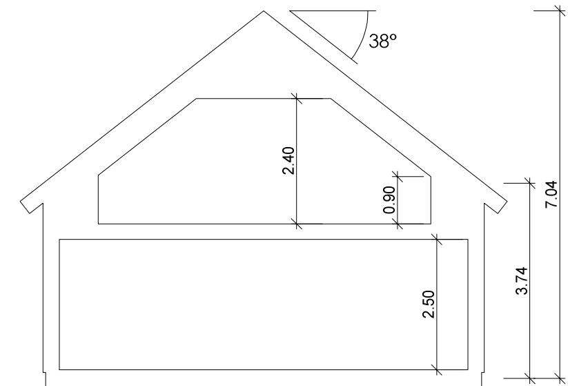
Sektion A-A
