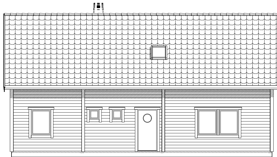
Fasad 1
