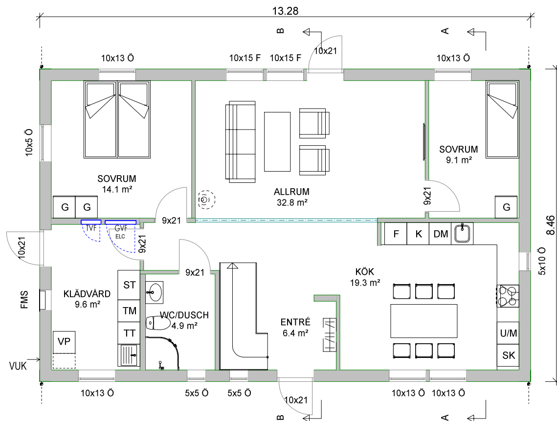
Entréplan BOA 99.1 m² BYA 112.3 m²
